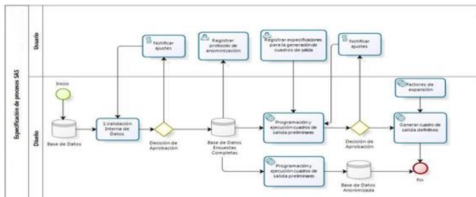
Figura 5. Especificación de procesos en SAS
