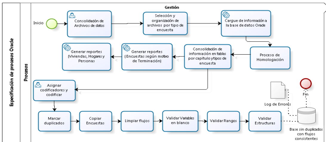
Figura 4. Especificación de procesos en Oracle
